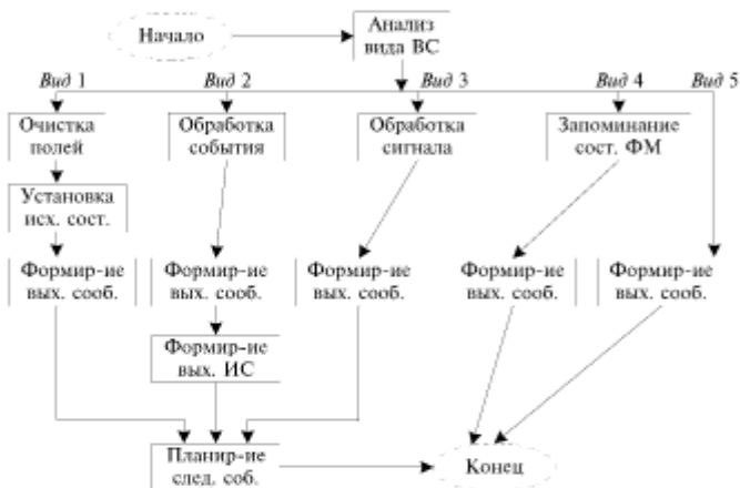
Рис. 11.8. Обобщенная блок-схема работы типового ФМ: ВС — входной сигнал; ИС — информационный сигнал
