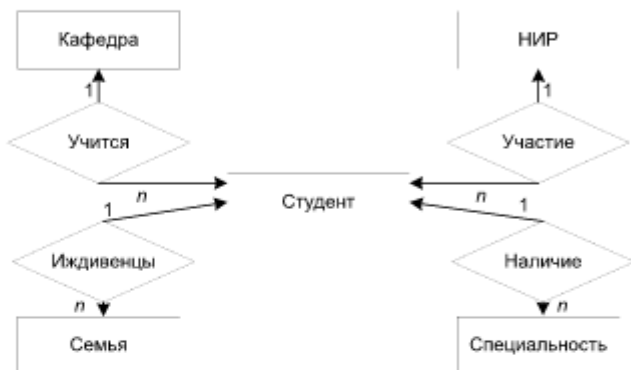
Рис. 7.5. Фрагмент ER-модели «Студенты»
