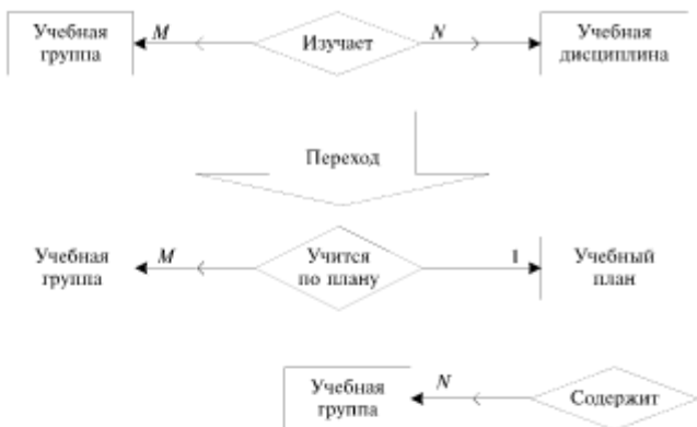
Рис. 7.8. Пример исключения связи типа M:N
