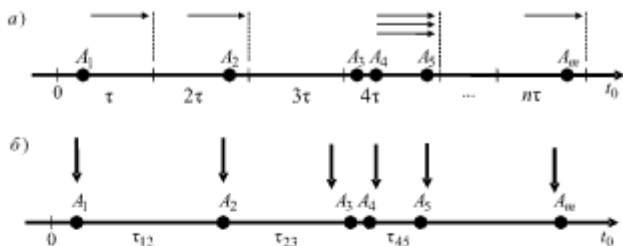
Рис. 11.2. Схемы реализации механизмов системного времени: а) с постоянным шагом; б) с переменным шагом
