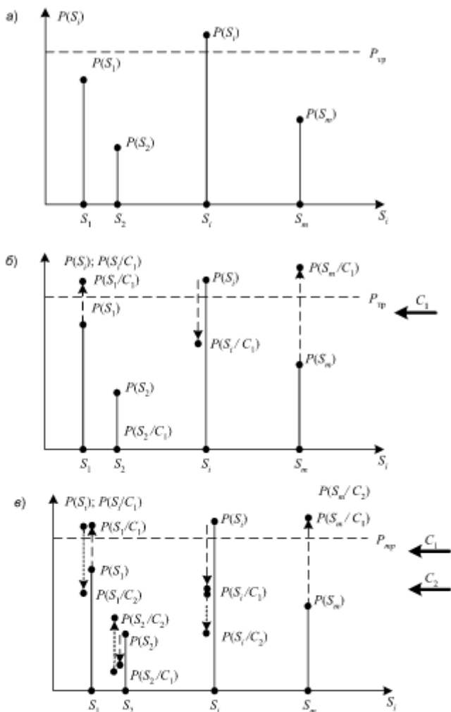
Рис. 17.8. Иллюстрация алгоритма работы диагностической ЭС Скопировано с сайта http://учебники.информ2000.рф Разработка электронных библиотек https://право.информ2000.рф
