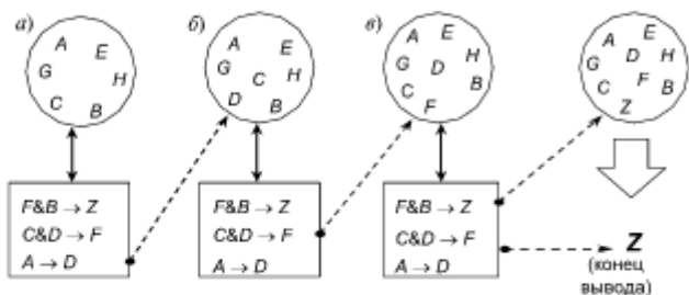
Рис. 17.1. Иллюстрация прямой цепочки рассуждений:
