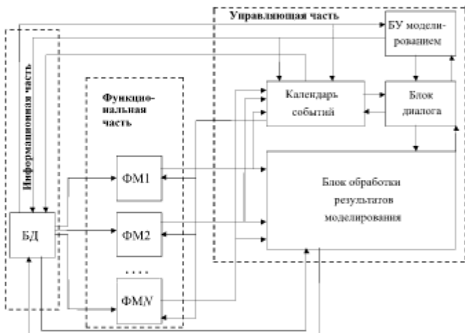
Рис. 11.5. Структура типовой имитационной модели с календарем событий
