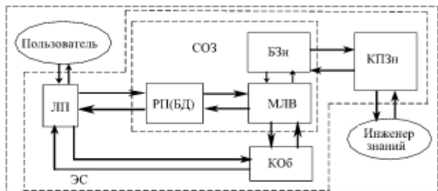
Рис. 16.1. Структура экспертной системы:
