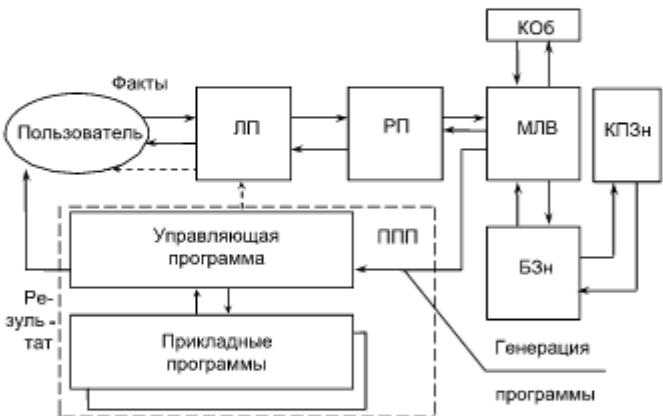
Рис. 16.2. Структура интеллектуального пакета прикладных программ
