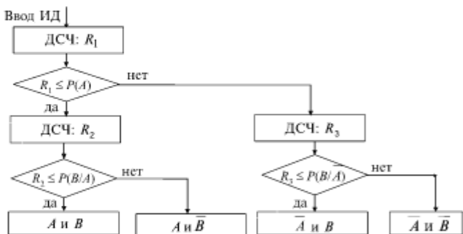
Рис. 12.7. «Последовательное моделирование» зависимых событий
