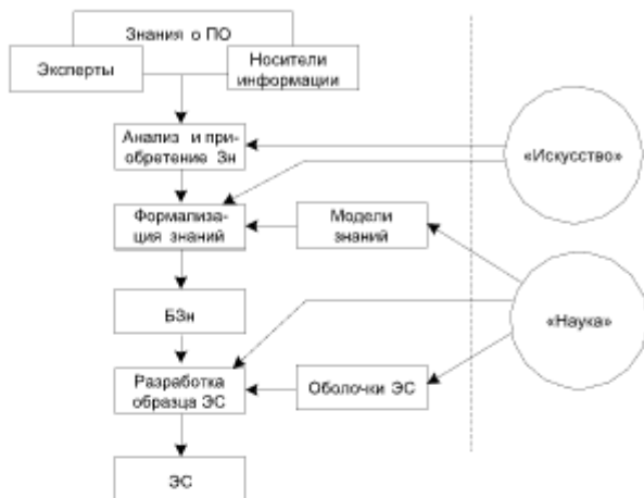
Рис. 16.5. Соотношение формальных и неформальных процедур при разработке ЭС
