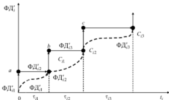
Рис 11.1. Схема моделирования функциональных действий в i -м компоненте системы
