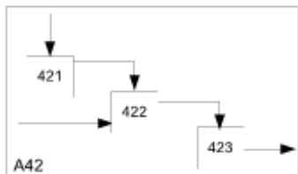
Рис. 6.2. Структура SADT-модели (декомпозиция диаграмм)
