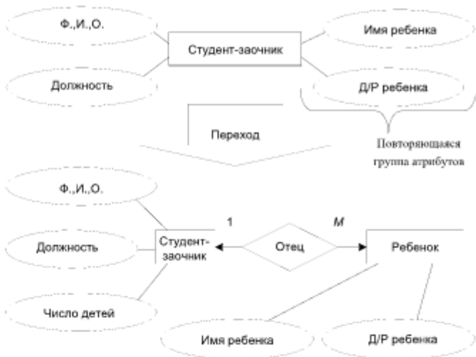
Рис 7.7. Пример исключения повторяющейся группы атрибутов
