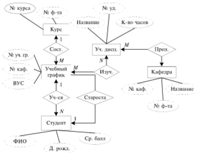
Рис. 7.6. Фрагмент ER-модели «Учебный процесс факультета»
