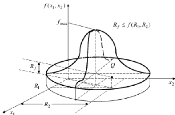
Рис. 12.14. Моделирование двумерного случайного вектора методом Неймана
