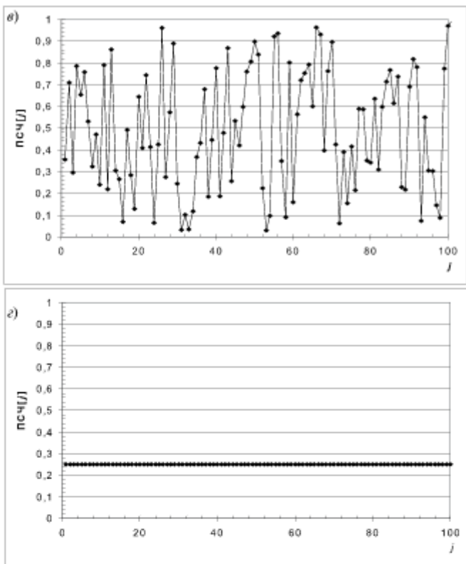
Рис. 12.1. Последовательности ПСЧ:
