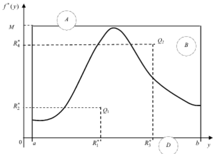
Рис. 12.11. Моделирование СВ методом Неймана
