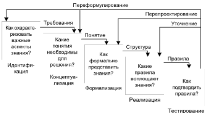
Рис. 16.6. Этапы разработки экспертной системы
