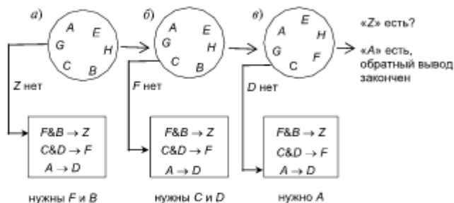
Рис. 17.2. Иллюстрация обратной цепочки рассуждений
