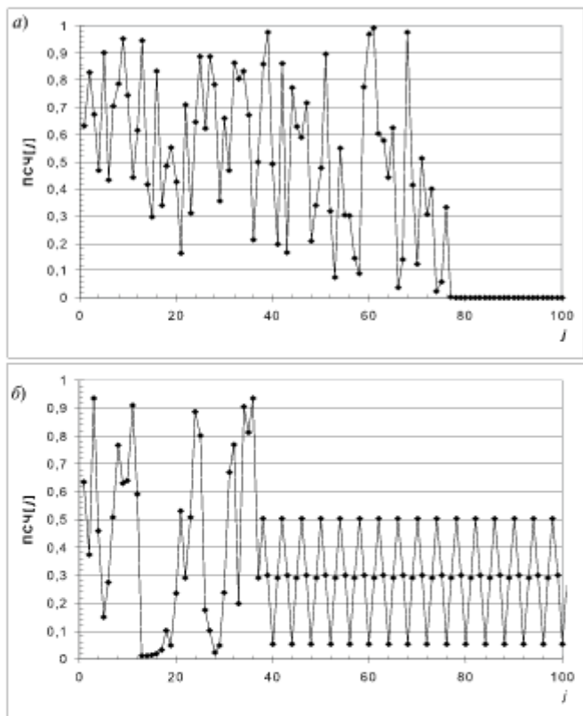
Рис. 12.1. Последовательности ПСЧ:
