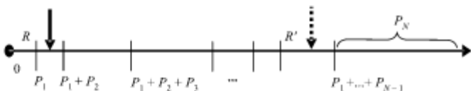
Рис. 12.13. Моделирование ДСВ методом последовательных сравнений
