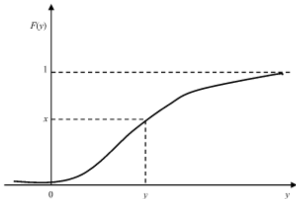
Рис. 12.10. Функция распределения СВ Y
