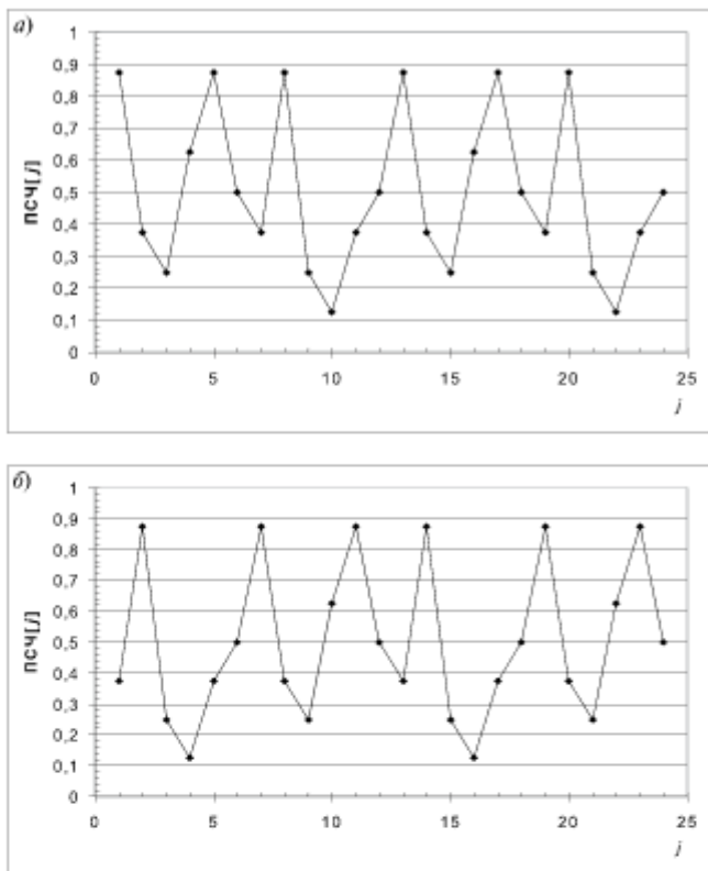
Рис. 12.3. Последовательности ПСЧ, полученные по аддитивному методу: а) X_0 = 1, X_1 = 3 ; б) X_0 = 5, X_1 = 7
