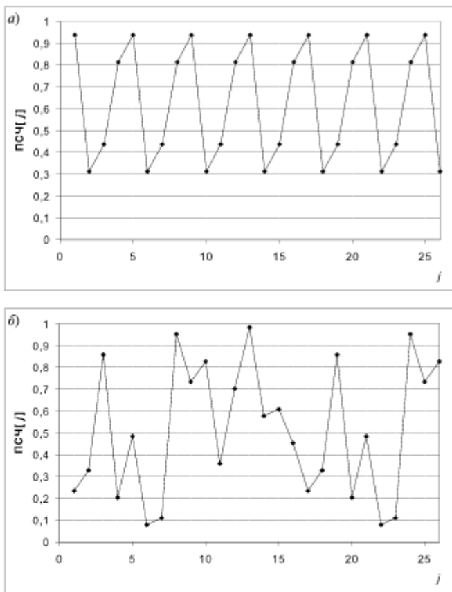
Рис. 12.2. Последовательности ПСЧ, полученные по мультипликативному методу:
