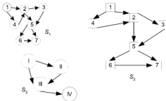
Рис. 10.3. Пример изоморфного и гомоморфного отображений: S_1 — система-оригинал; S_2 — изоморфное отображение оригинала; S_3 — гомоморфное отображение оригинала.
