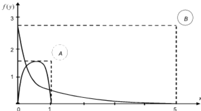
Рис. 12.12. Иллюстрация результатов оценки эффективности метода Неймана
