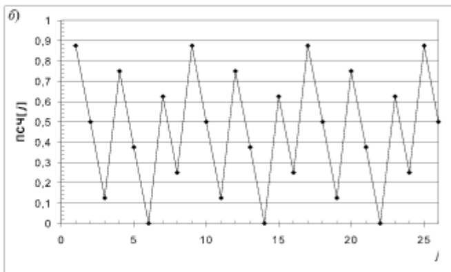
Рис. 12.4. Последовательности ПСЧ, полученные по смешанному методу: а) b = 3 ; б) b = 4
