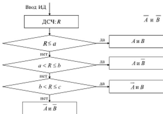
Рис. 12.9. Алгоритм моделирования зависимых случайных событий «после предварительных расчетов»
