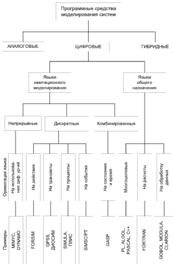
Рис. 13.3. Классификация программных средств моделирования систем
